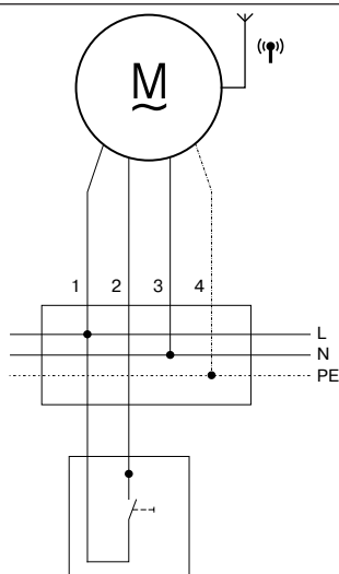
Tlačítko (uzavírací)
